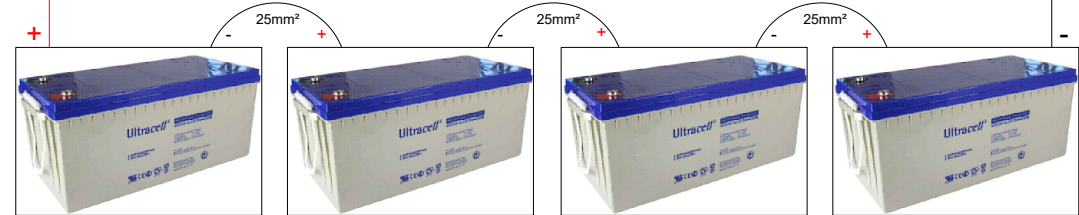
Batterie 12V
